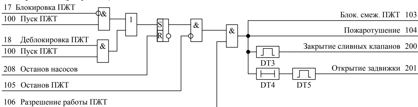
Рисунок 8 – Ввод в работу пожаротушения
