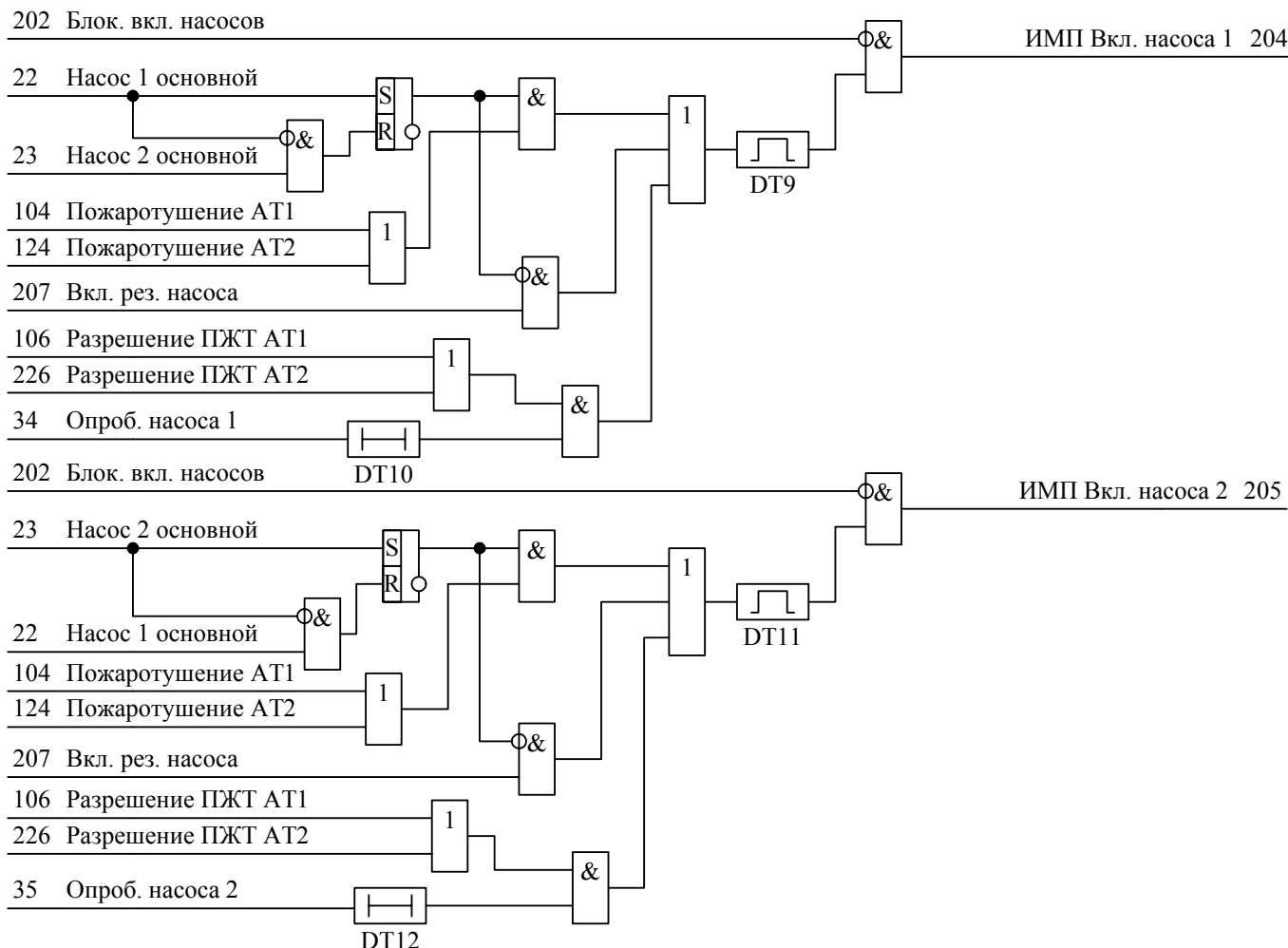
Рисунок 24 – Управление насосами
