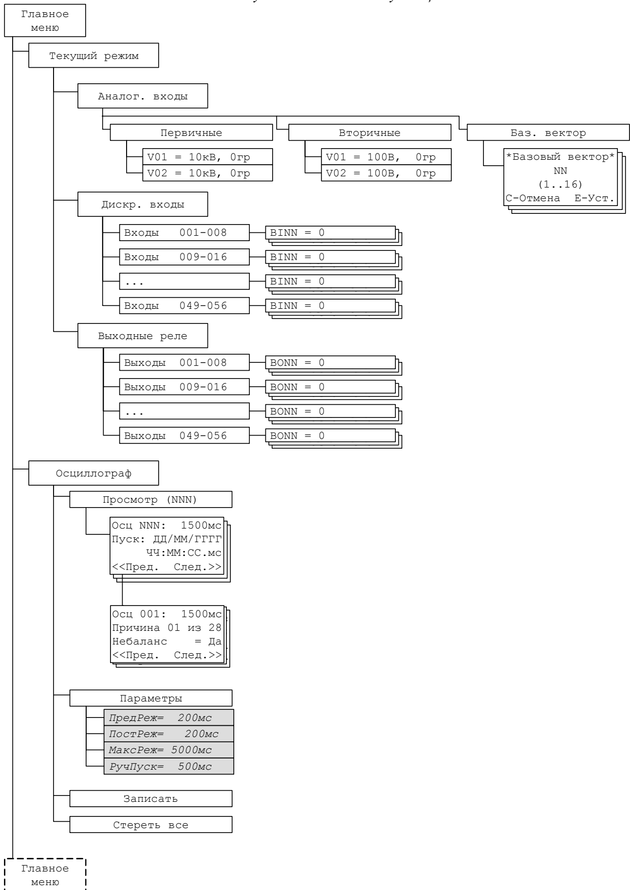
Рисунок 46 – Дерево меню (Текущий режим, Осциллограф)
