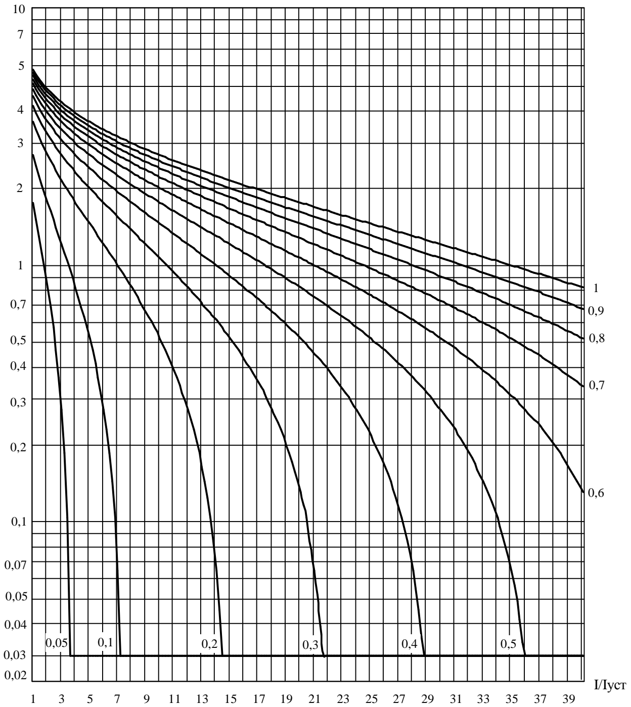
Рис.3.3.5.5 – Характеристика RXIDG-типа
